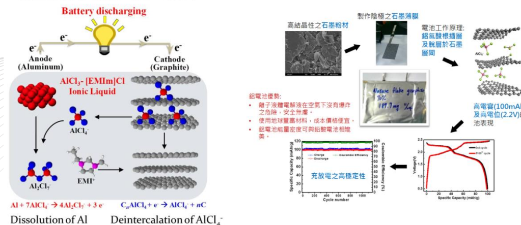
可充放電鋁離子電池之工作原理示意圖
